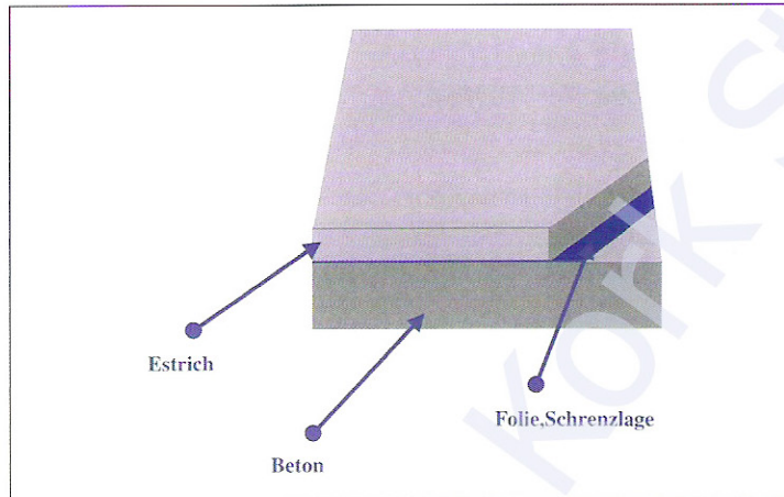
Konstruktionsaufbau Estrich auf Trennlage nach DIN 18560 Teil 3
