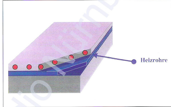
Konstruktionsaufbau Verbundestrich nach DIN 18560 Teil 4
